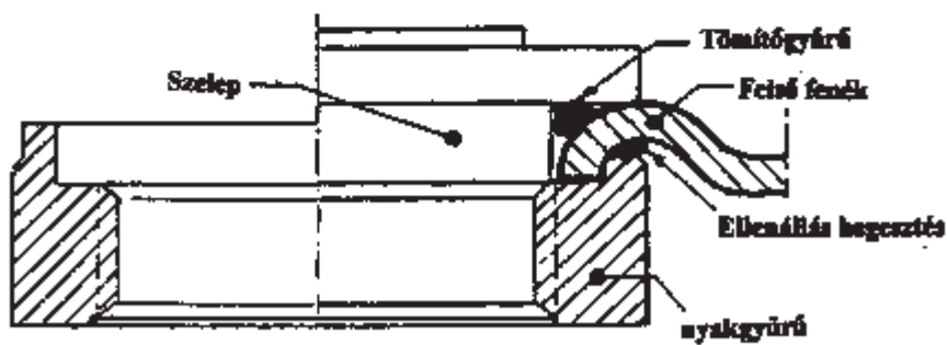
4. ábra A betűl elhelyezett nyakgyűrű hegesztési varrata
